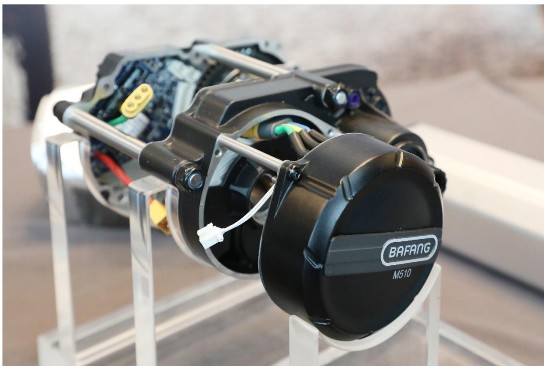
八方 M510 电机爆炸模型
